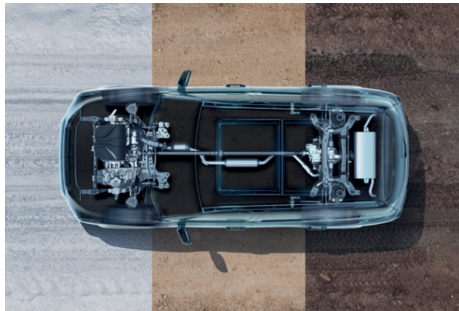
Интеллектуальный полный привод и 8 режимов вождения
