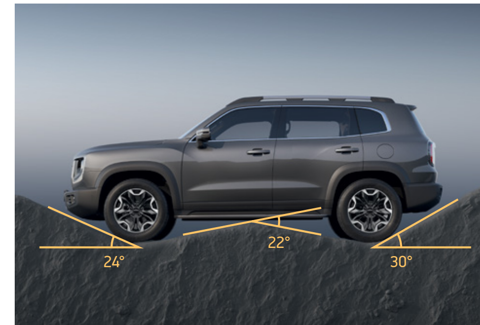
Углы въезда, рампы и съезда
